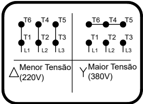
Fechamento para Motobombas trifásicas
