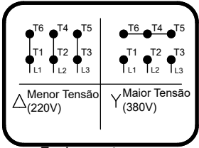
Fechamento para Motobombas trifásicas
