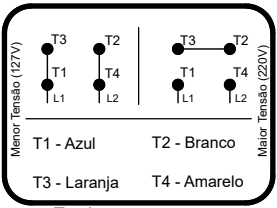
Fechamento para Motobombas monofásicas
