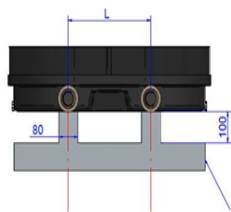
Fig. 2 Instalação em base de hormigón com elevação.
