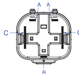
Fig. 4 - Posições de montagem de los calzos de amortiguación
