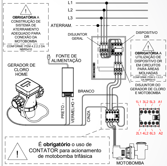
Ligação do Gerador de Cloro Easyclor Home em rede elétrica trifásica 220 VCA
