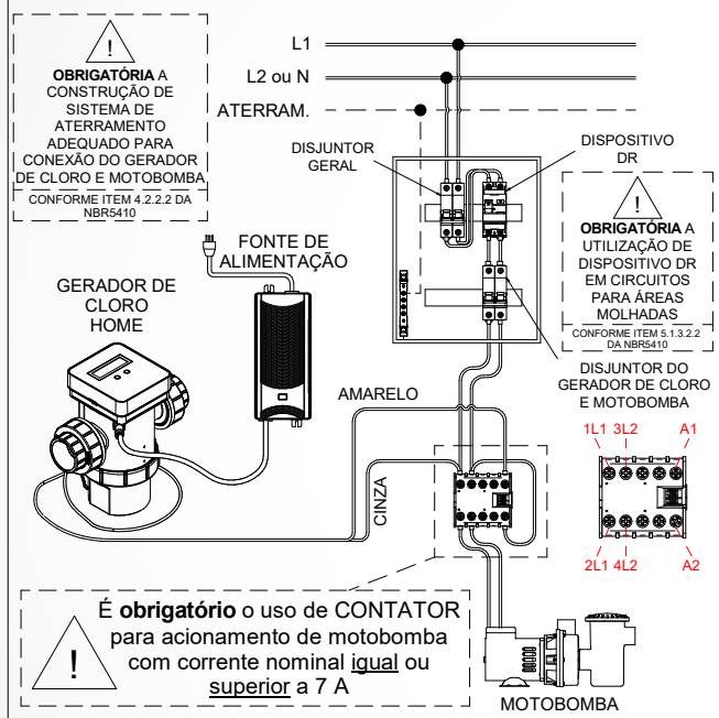
Ligação do Gerador de Cloro Easyclor Home em rede elétrica monofásica 127 VCA e 220 VCA
