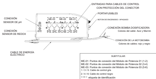
VISTA INFERIOR DEL MÓDULO DE CONTROL
