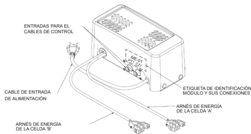
VISTA ISOMÉTRICA DEL MÓDULO DE POTENCIA
