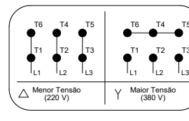
Fechamento para Motobombas Trifásicas
