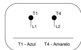
Fechamento para Motobombas Monofásicas 127 V ou 220 V
