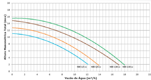
CURVA CARACTERÍSTICA NBE TRIFÁSICA
