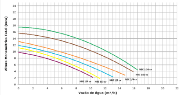
CURVA CARACTERÍSTICA NBE MONOFÁSICA
