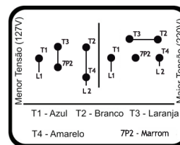
Fechamento para motobombas monofásicas
